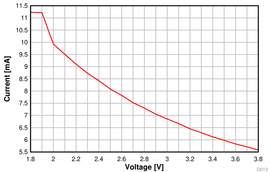
RX Current vs. VDD5 BLE 1 Mbps, 2.44 GHz
